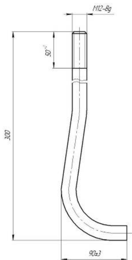
Болт фундаментный АЗТ 8.926.002
