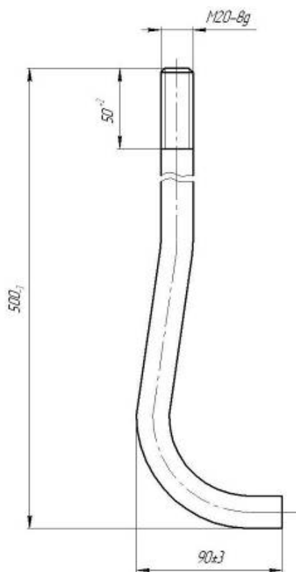
Болт фундаментный 3Ш8.926.046
