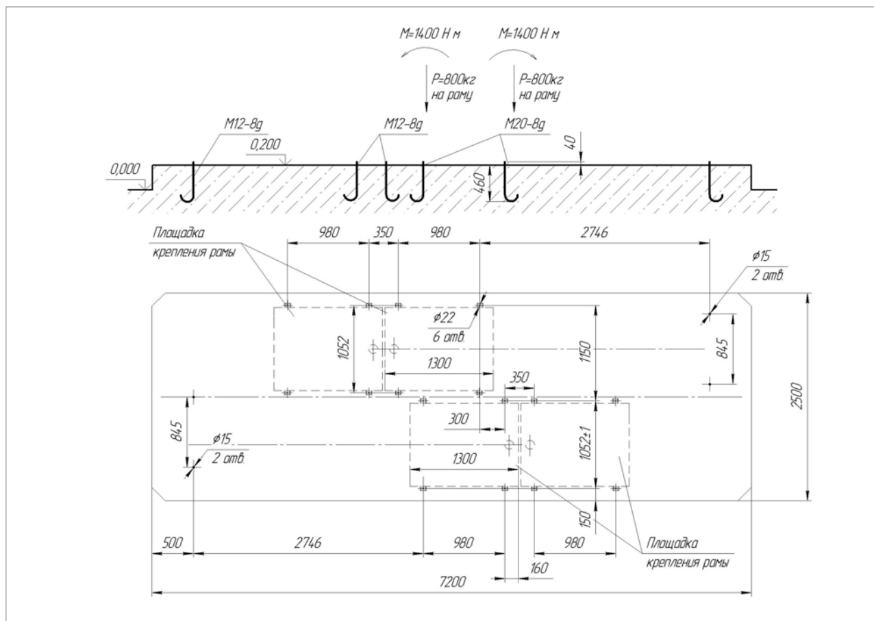
Комплекс измерительный АСН-10ВГ модуль Ду100 2/4 без насоса. План фундаментов.
