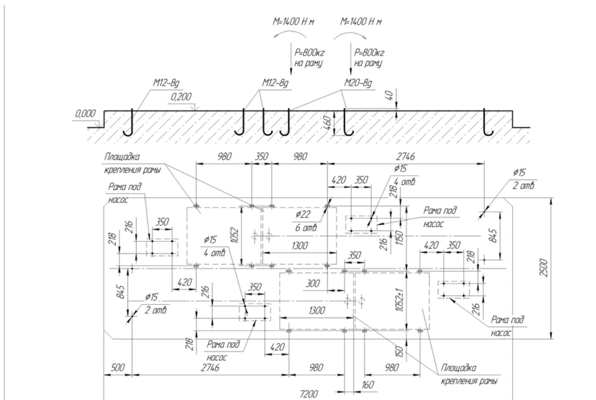
Комплекс измерительный АСН-10ВГ модуль Ду100 2/4 с насосами КМ и КМС. План фундаментов.
