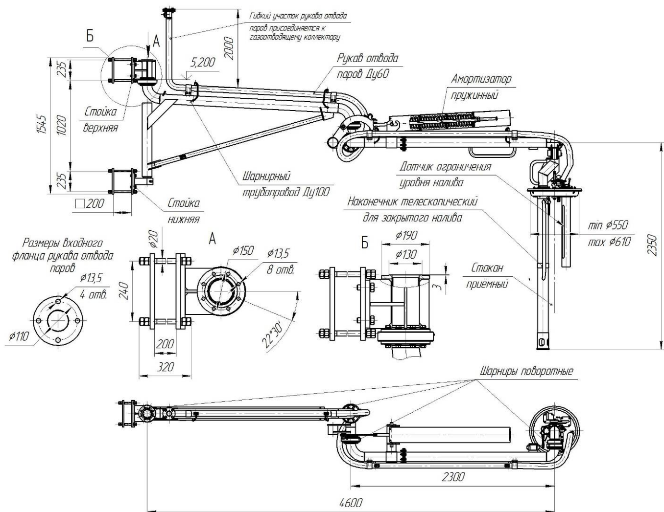
Рисунок 1.2 – Стояк наливной АСН-14ЖД-К правое исполнение.
