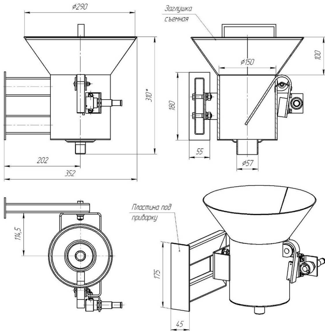
Рисунок 1.4 – Габаритные размеры стационарного каплесборника, устанавливаемого на металлоконструкции (поставляется по доп. заказу).
