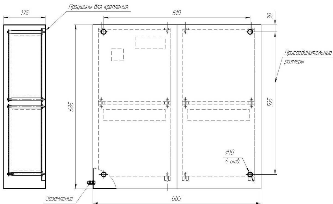
Рисунок 1.4 – Габаритные размеры стационарного каплесборника, устанавливаемого на металлоконструкции (поставляется по доп. заказу).
