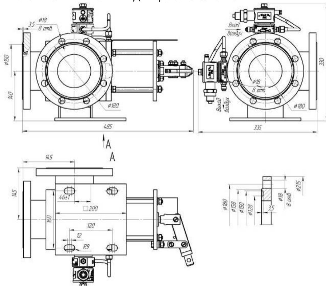
Рисунок 1.3 – Клапан отсекающий КО.
